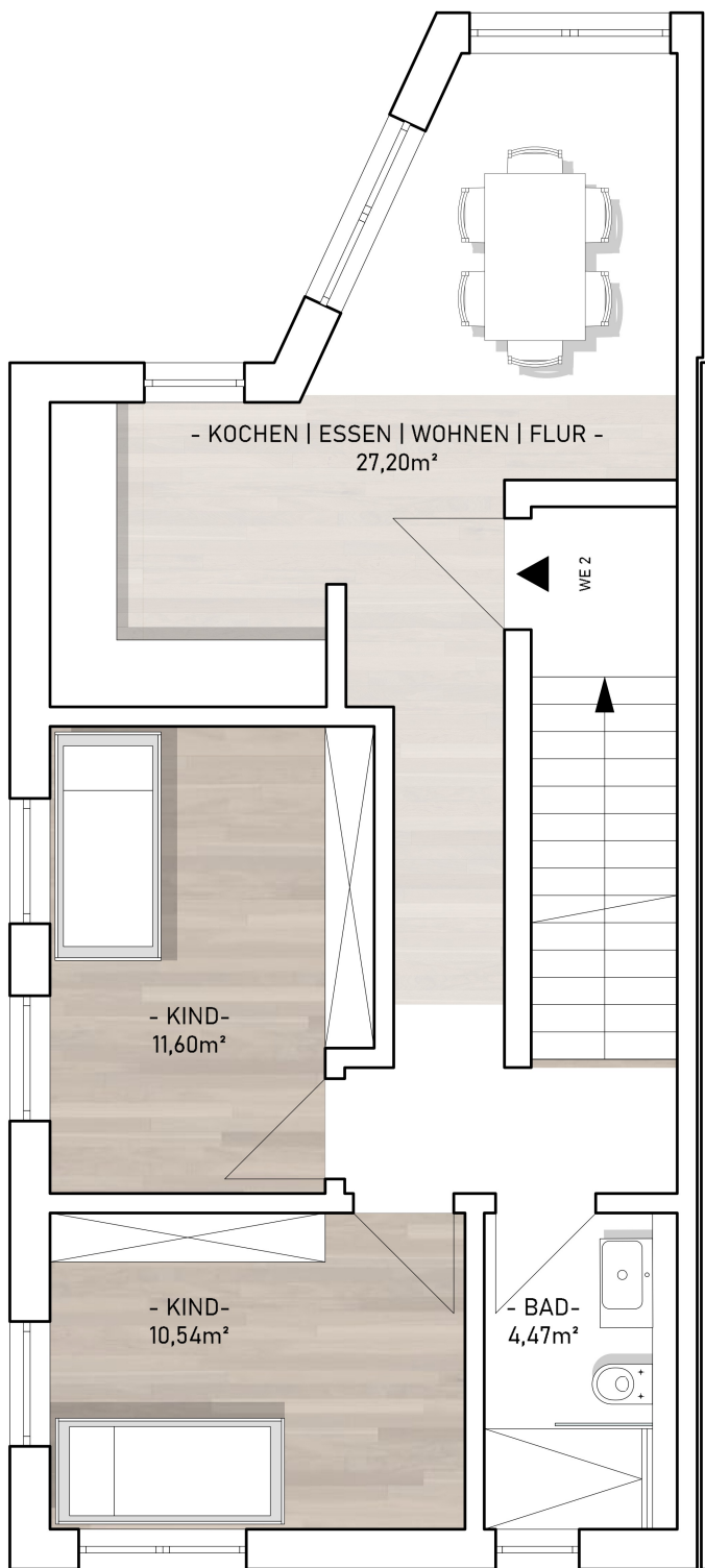
I. OBERGESCHOSS
